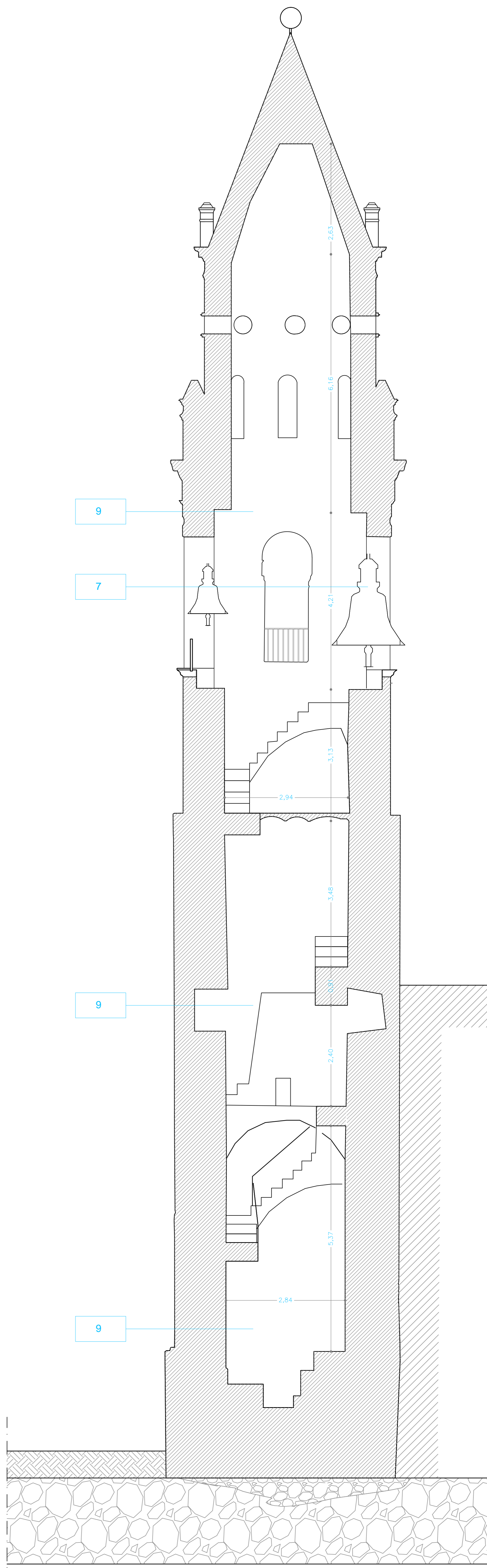
SEZIONE A-A' SCALA 1:100
